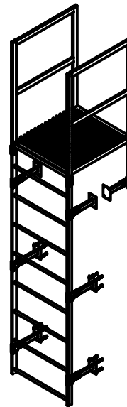
Вертикальная пожарная лестница П1-1 PP ROLLED
