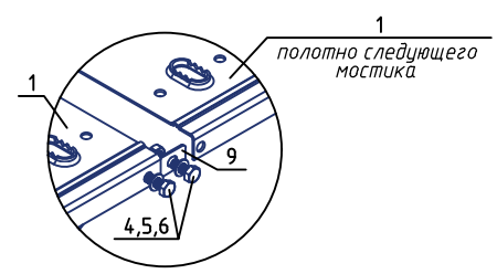
Соединение полотен
