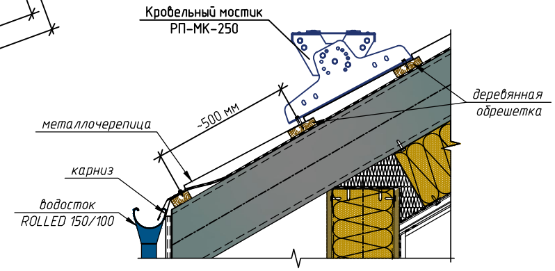
Типовой узел крепления кровельного мостика РП-МК-250 на металлочерепицу
