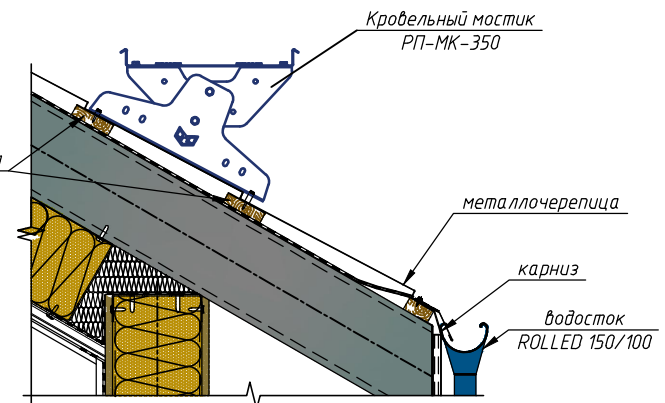
Типовой узел крепления кровельного мостика РП-МК-350 на металлочерепицу
