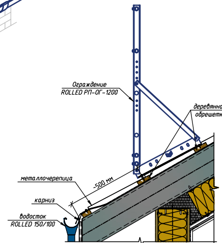
Типовой узел крепления ограждения на металлочерепицу
