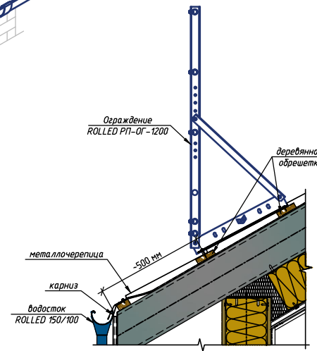
Типовой узел крепления ограждения на металлочерепицу
