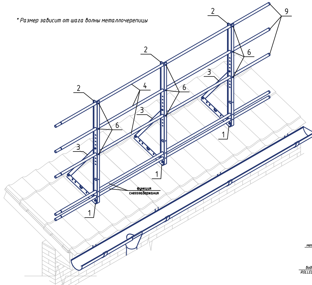
Типовой узел крепления ограждения на металлочерепицу
