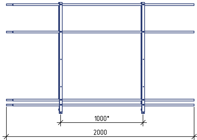
Ограждение ROLLED+ 1200 (l=2000 мм) +ФС
