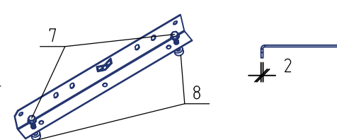
Сечение опорной стойки 1200 ROLLED+
