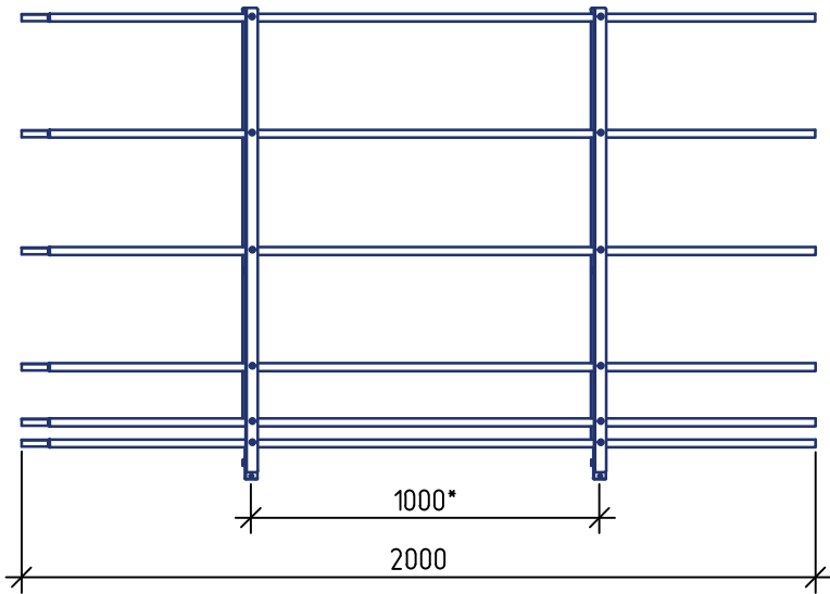
Ограждение ROLLED+ 1200 (l=2000 мм) -2ДТ+ФС
