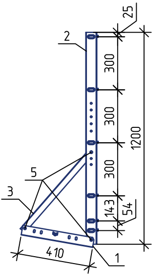
Вид А
