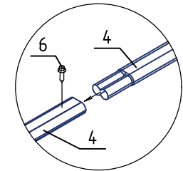
Узел крепления к кровле
