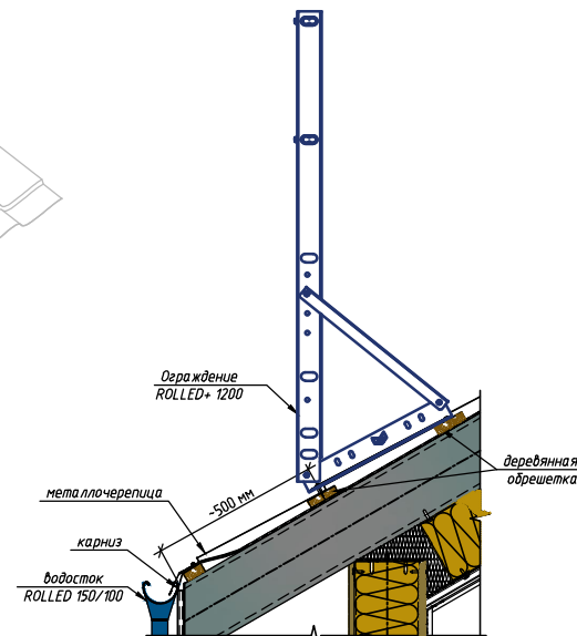
Типовой узел крепления ограждения на металлочерепицу
