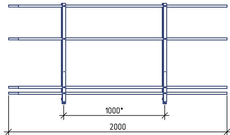
Ограждение ROLLED+ 900 (l=2000 мм)+ФС
