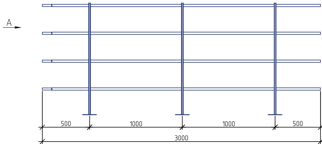
Ограждение РП-ОГ-ПР-1200 (l=3000 мм) -2ДТ (общий вид)
