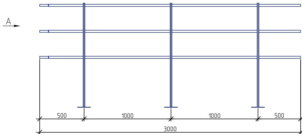
Ограждение РП-ОГ-ПР-1200 (l=3000 мм) - ДТ (общий вид)
