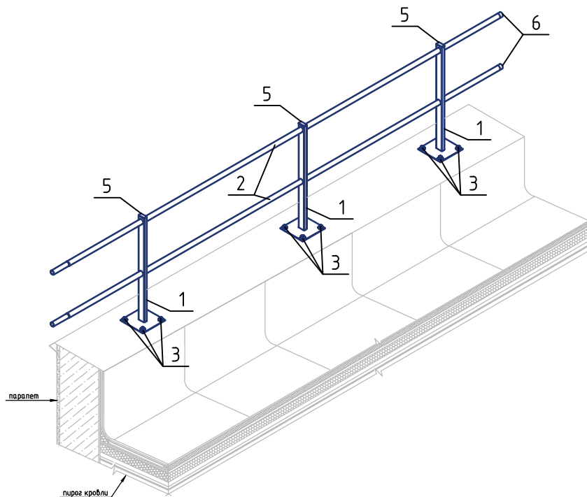
Ограждение РП-ОГ-ПР-600 (l=3000 мм) (общий вид)
