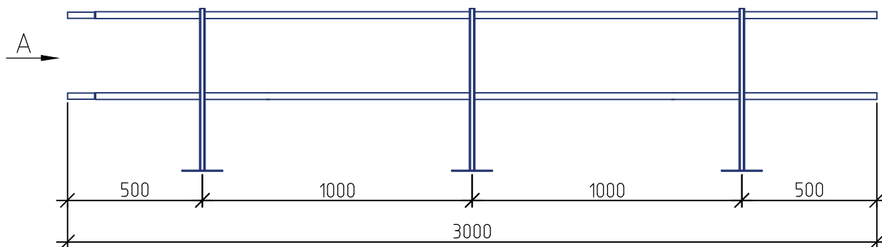
Ограждение РП-ОГ-ПР-600 (l=3000 мм)
