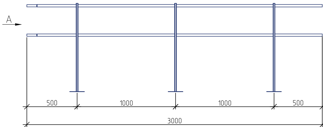
Ограждение РП-ОГ-ПР-900 (l=3000 мм) (общий вид)
