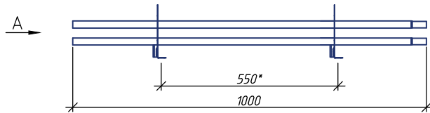
Снегозадержатель РПФ-40_20 (2 опоры)
