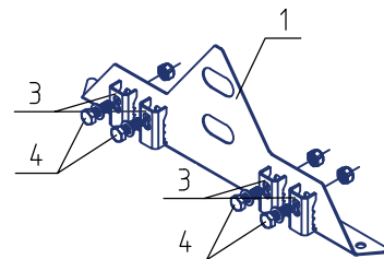
Опора РП-Овал в сборе
