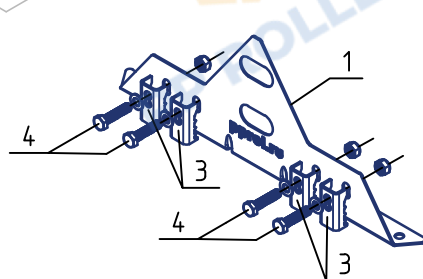
Крепление опоры
