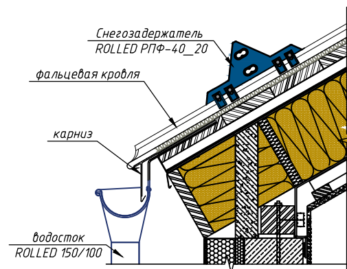
Типовой узел крепления снегозадержателя на фальцевую кровлю
