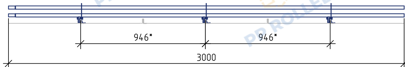
Вид сбоку
