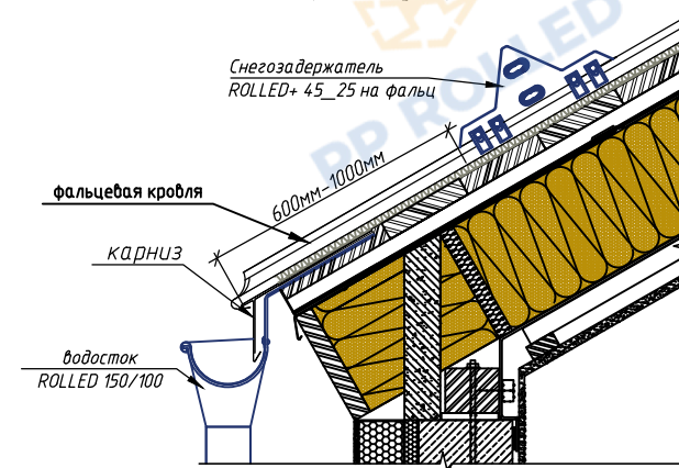
Типовой узел крепления снегозадержателя на фальцевую кровлю
