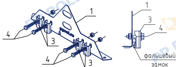
Крепление опоры
