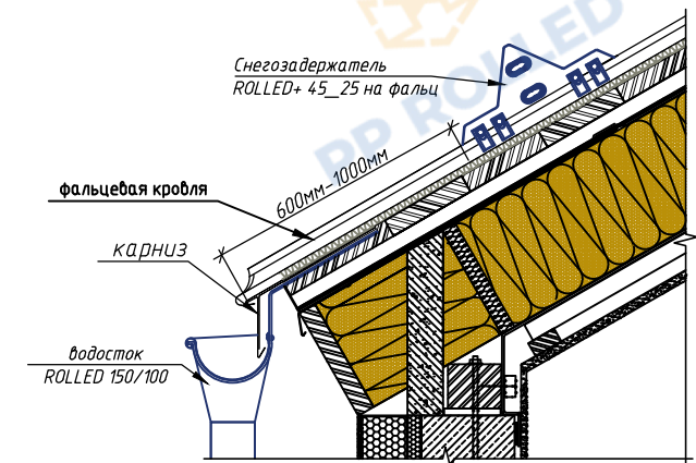
Типовой узел крепления снегозадержателя на фальцевую кровлю
