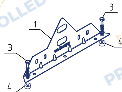
Крепление опоры
