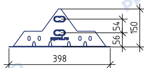
Вид сбоку
