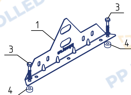
Крепление опоры
