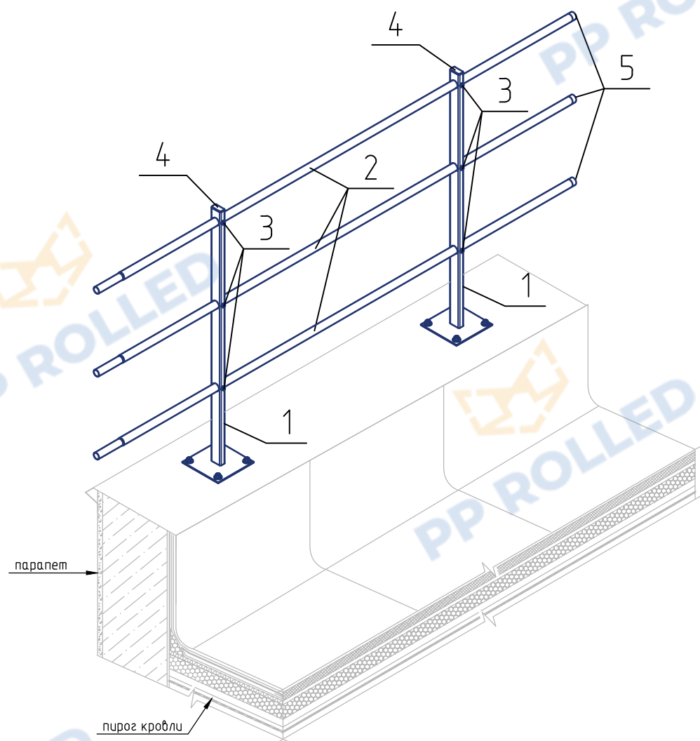
Ограждение РП-ОГ-ПР-900 (l=2000 мм)-ДТ (общий вид)
