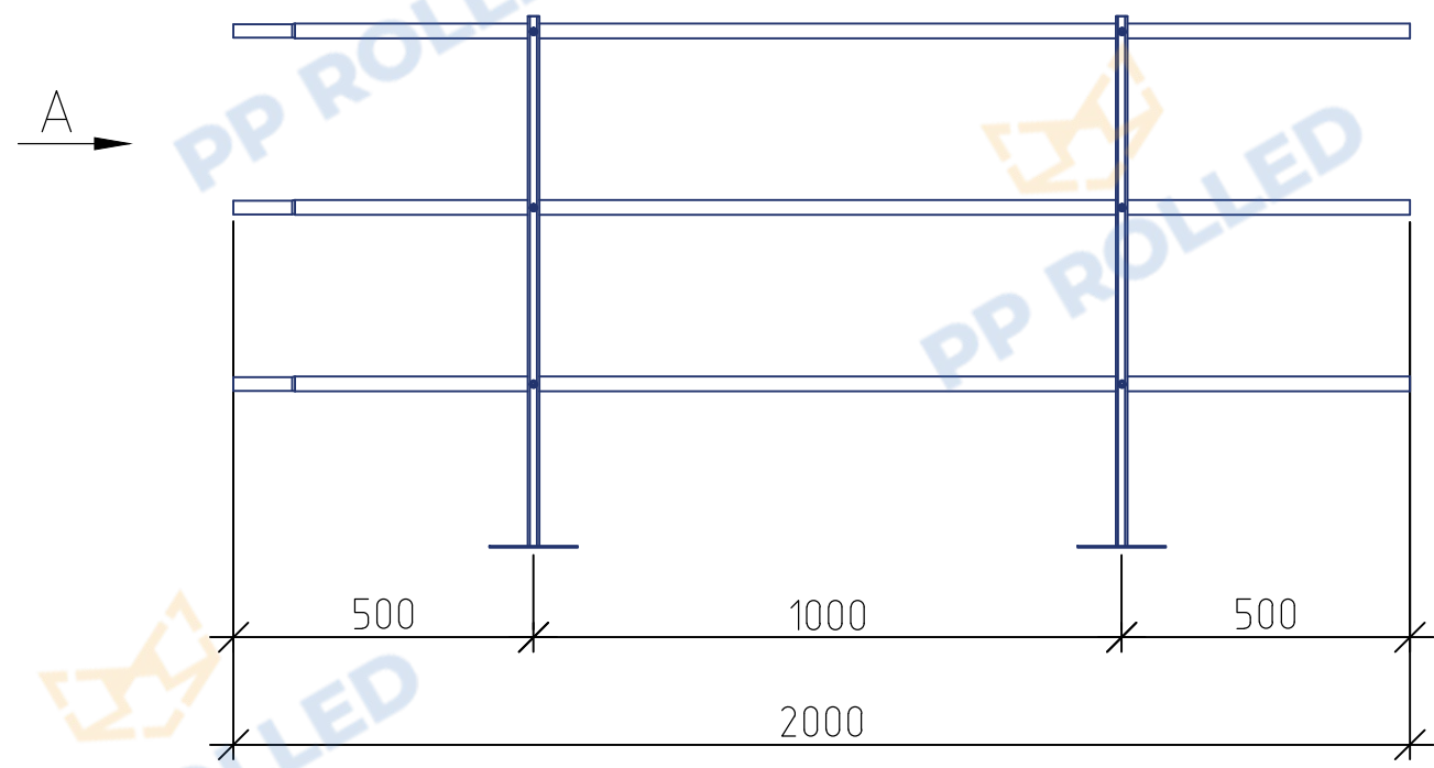
Ограждение РП-ОГ-ПР-900 (l=2000 мм) PP ROLLED
