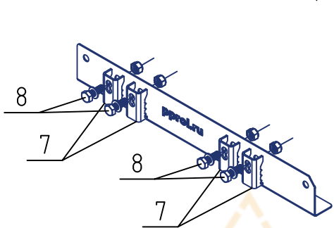
Опора РП-ОГ в сборе
