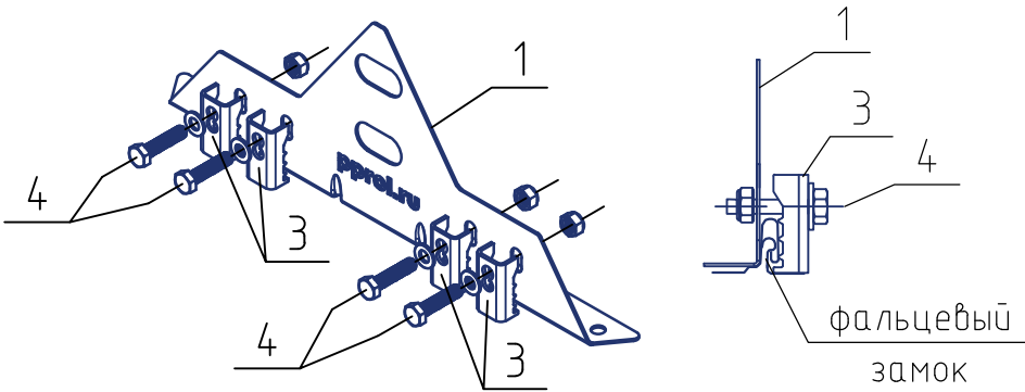
Крепление опоры
