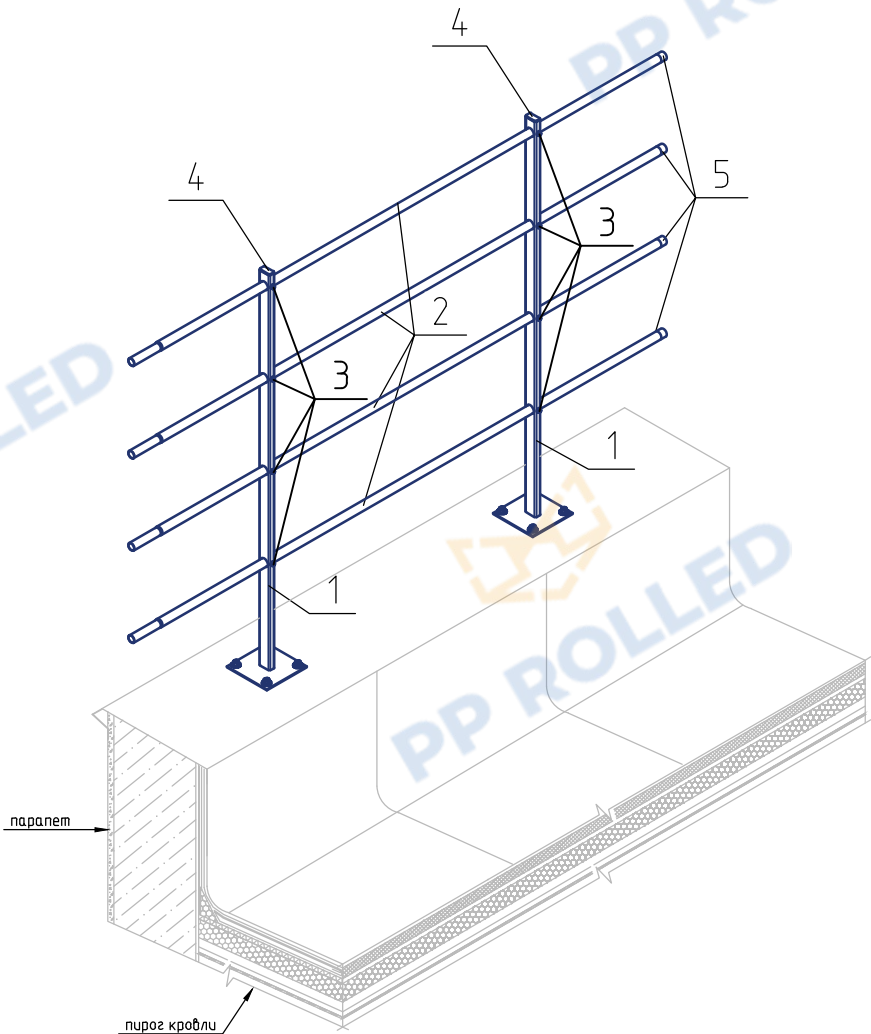
Ограждение РП-ОГ-ПР-1200 (l=2000 мм) -2ДТ (общий вид)
