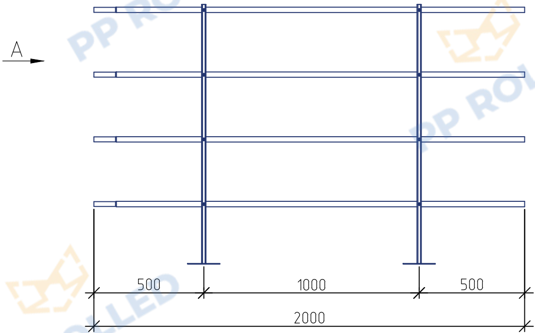
Ограждение РП-ОГ-ПР-1200 (l=2000 мм) -2ДТ (общий вид)
