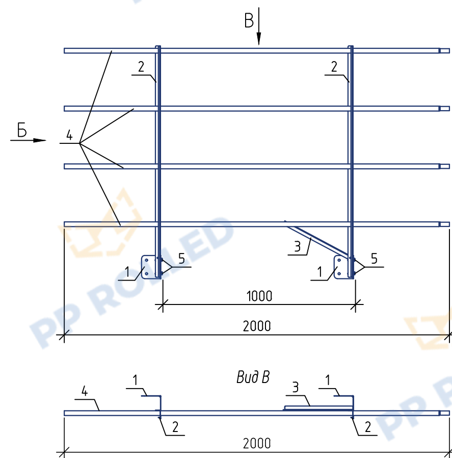
Ограждение РП-ДЕК-ПРС-1200 (l=2000 мм) PP ROLLED Вариант 2 (крепление сбоку парапета)
