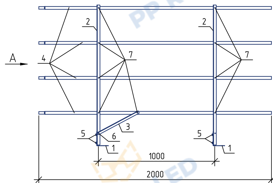
Ограждение РП-ДЕК-ПРС-1200 (l=2000 мм) PP ROLLED Вариант 2 (крепление сбоку парапета)
