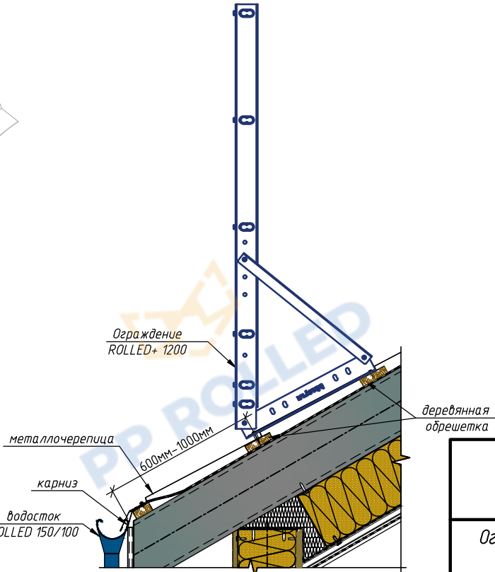
Типовой узел крепления ограждения на металлочерепицу
