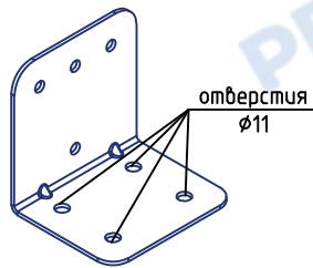
Опора РП-ПРС
