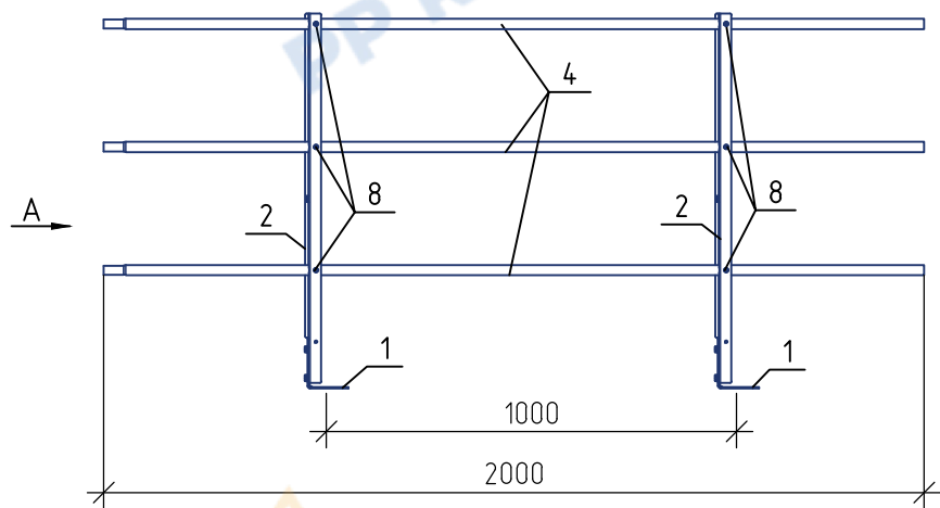
Ограждение РП-ПРС-900 (l=2000 мм) PP ROLLED Вариант 2 (крепление сбоку парапета)
