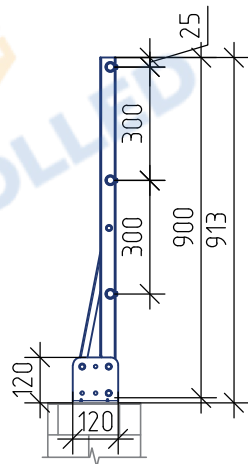
Вид А
