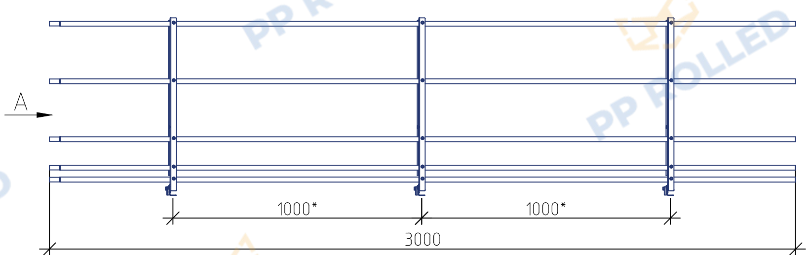
Ограждение РПФ-ОГ-900 (l=3000мм)+ФЦ PP ROLLED
