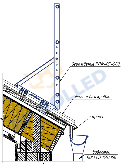
Типовой узел крепления ограждения на фальцевую кровлю
