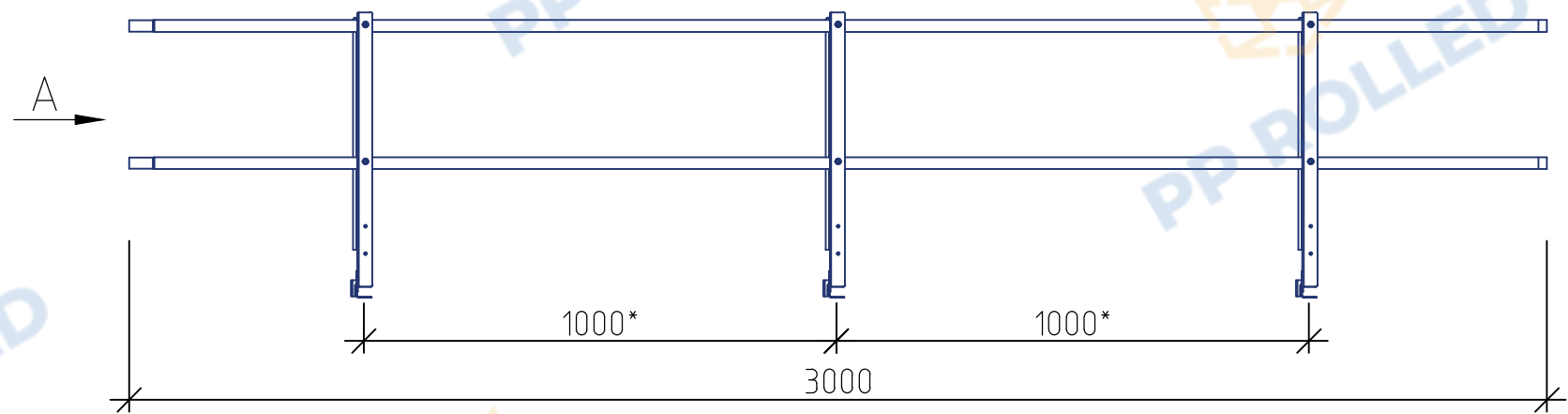
Ограждение РПФ-ОГ-600 (l=3000 мм) PP ROLLED
