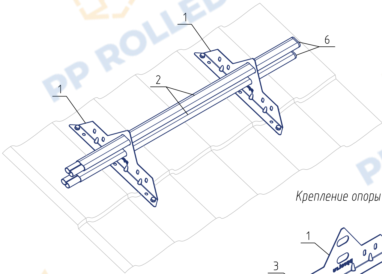
Общий вид
