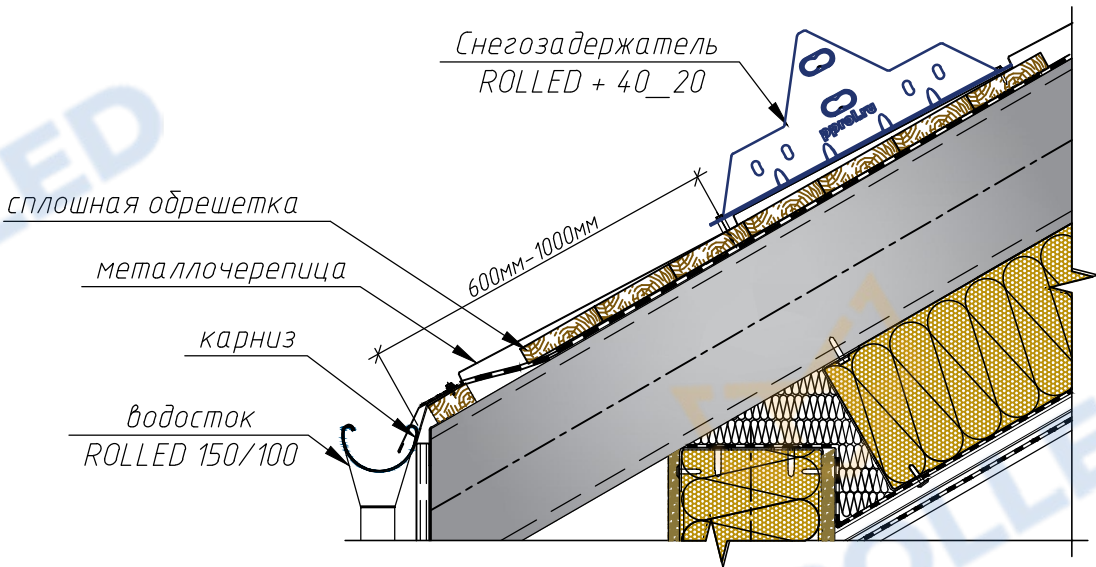
Типовой узел крепления снегозадержателя на металлочерепицу
