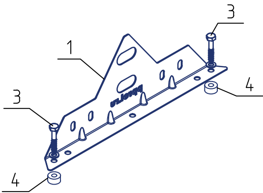
Крепление опоры
