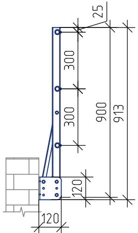
Вид Б
