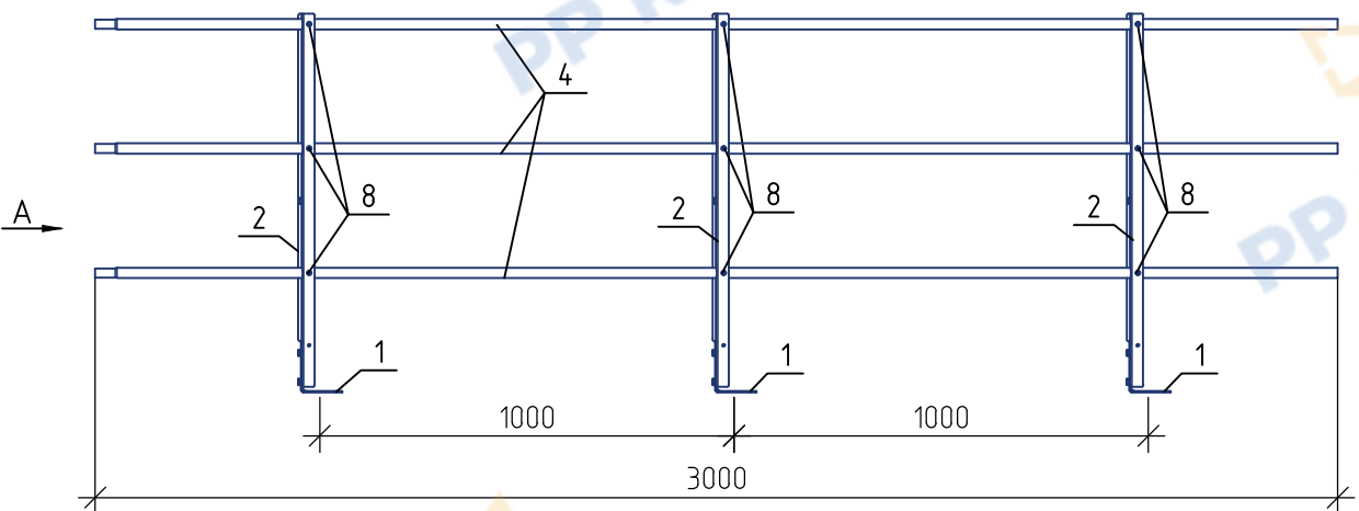
Ограждение РП-ПРС-900 (L=3000 мм) PP ROLLED Вариант 2 (крепление сбоку парапета)
