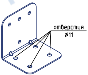
Опора РП-ПРС
