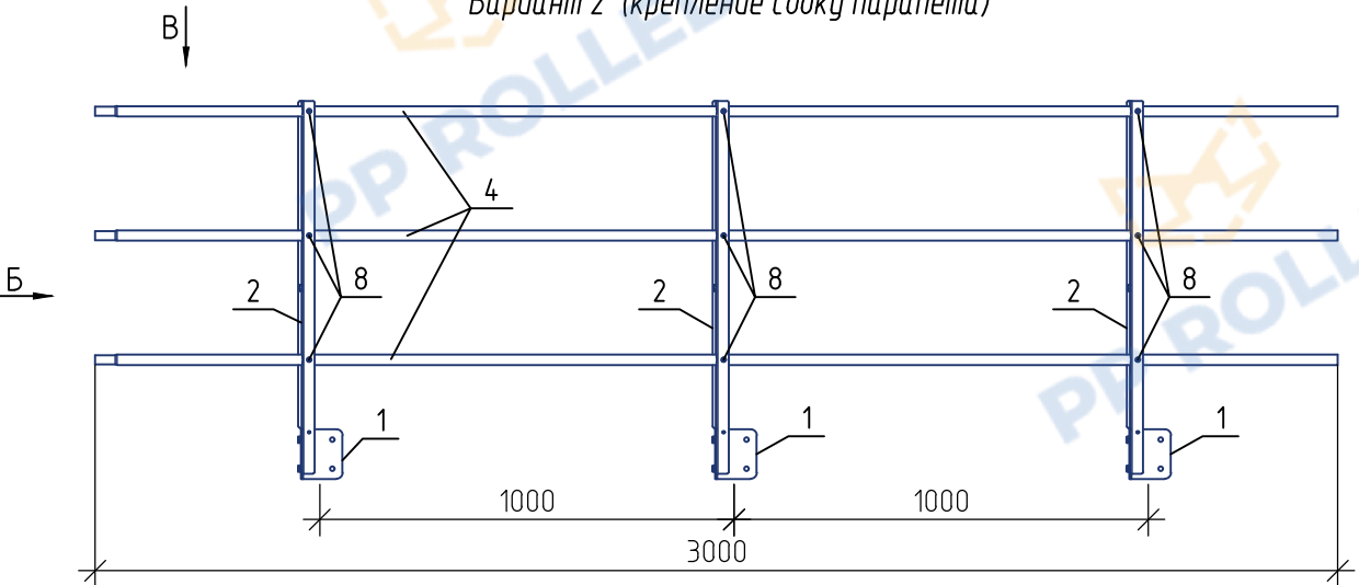
Ограждение РП-ПРС-900 (L=3000 мм) PP ROLLED Вариант 2 (крепление сбоку парапета)
