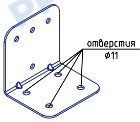
Опора РП-ПРС
