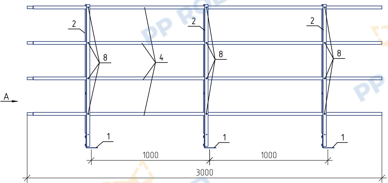
Ограждение РП-ПРС-1200 (l=3000 мм) PP ROLLED Вариант 2 (крепление сбоку парапета)
