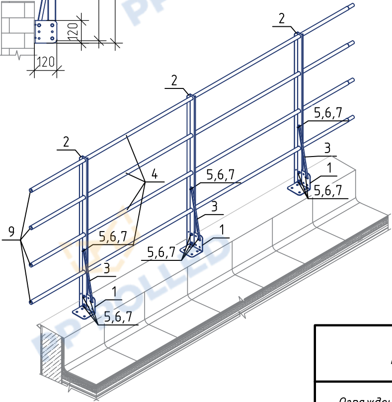
Общий вид (вариант 1)
