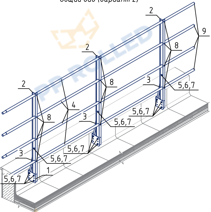
Общий вид (вариант 2)
