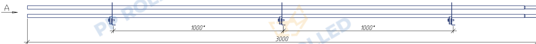
Опора РП-СН-40х20 в сборе
