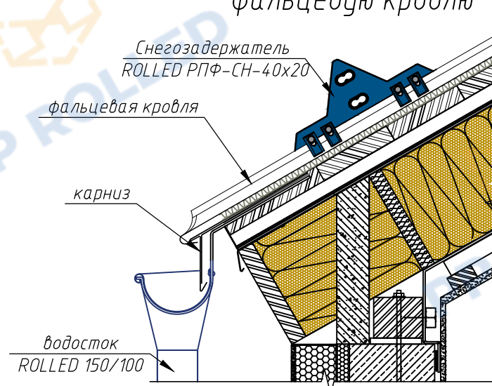
Типовой узел крепления снегозадержателя на фальцевую кровлю
