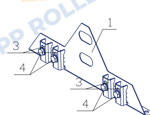
Опора РП-СН-40х20 в сборе
