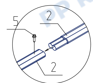
Узел крепления труб
