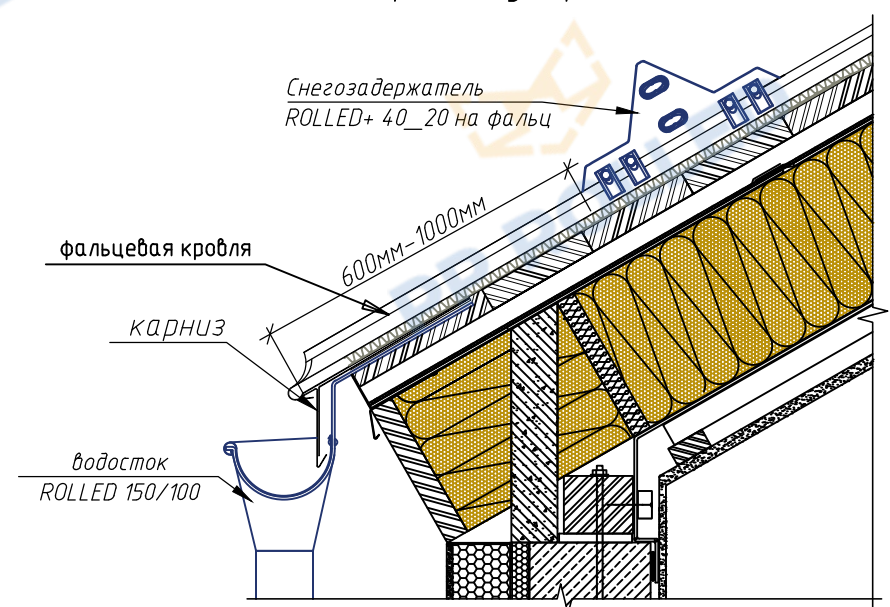
Типовой узел крепления снегозадержателя на фальцевую кровлю
