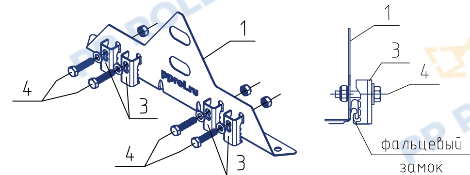
Крепление опоры
