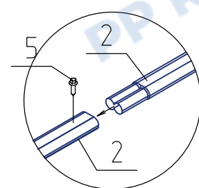
Узел крепления труб
