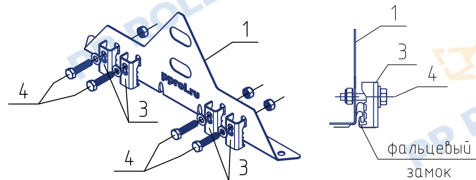
Крепление опоры
