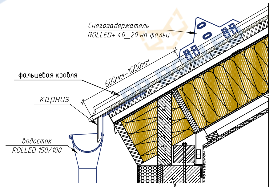
Типовой узел крепления снегозадержателя на фальцевую кровлю
