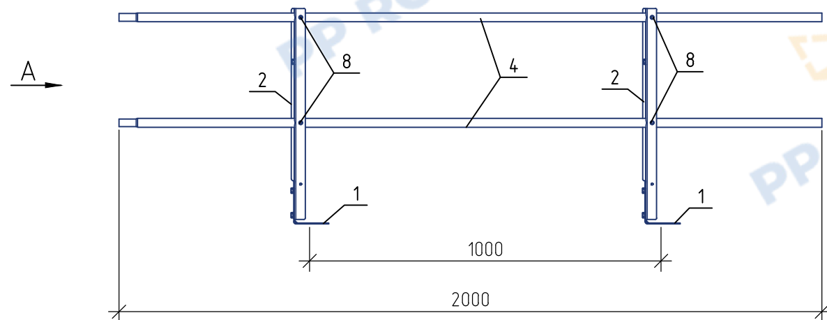
Ограждение РП-ПРС-600 (l=2000 мм) PP ROLLED Вариант 2 (крепление сбоку парапета)
