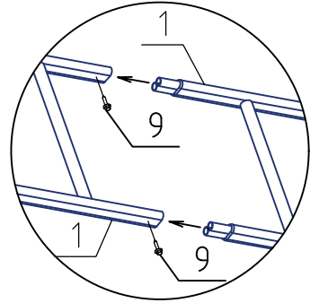
Узел соединения лестничных полотен
