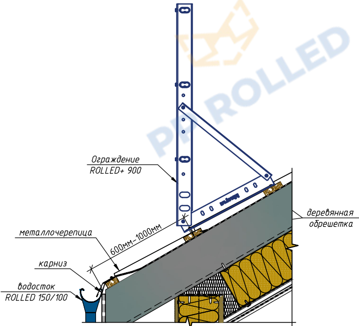
Типовой узел крепления ограждения на металлочерепицу
