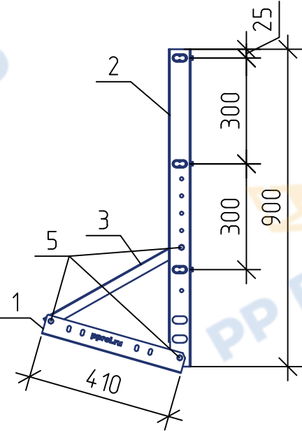
Вид А
