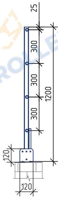
Вид Б
