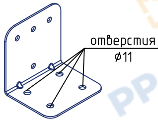
Опора РП-ДЕК-ПРС
