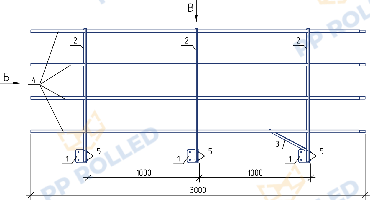
Ограждение РП-ДЕК-ПРС-1200 (l=3000 мм) PP ROLLED Вариант 2 (крепление сбоку паралета)
