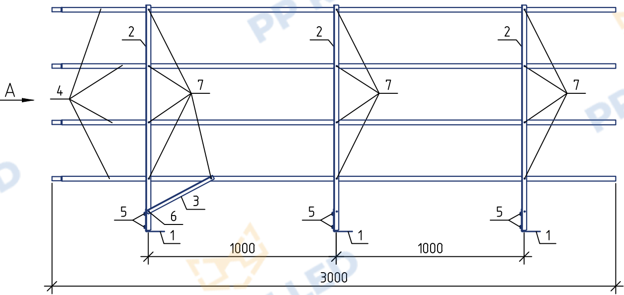
Ограждение РП-ДЕК-ПРС-1200 (l=3000 мм) PP ROLLED Вариант 2 (крепление сбоку паралета)
