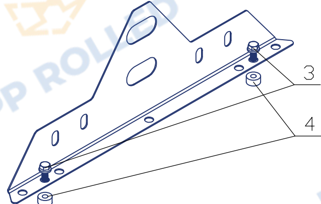
Опора РП-СН-40х20
