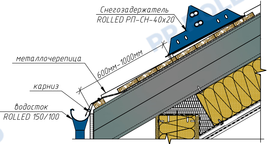
Типовой узел крепления снегозадержателя на металлочерепицу
