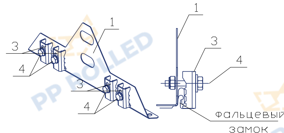
Опора РП-СН-40х20 в сдоре
