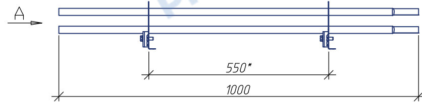
Снегозадержатель РП-СН-40х20-1,5 (2 опоры) на фальц
