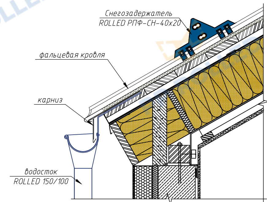
Типовой узел крепления снегозадержателя на фальцевую кровлю
