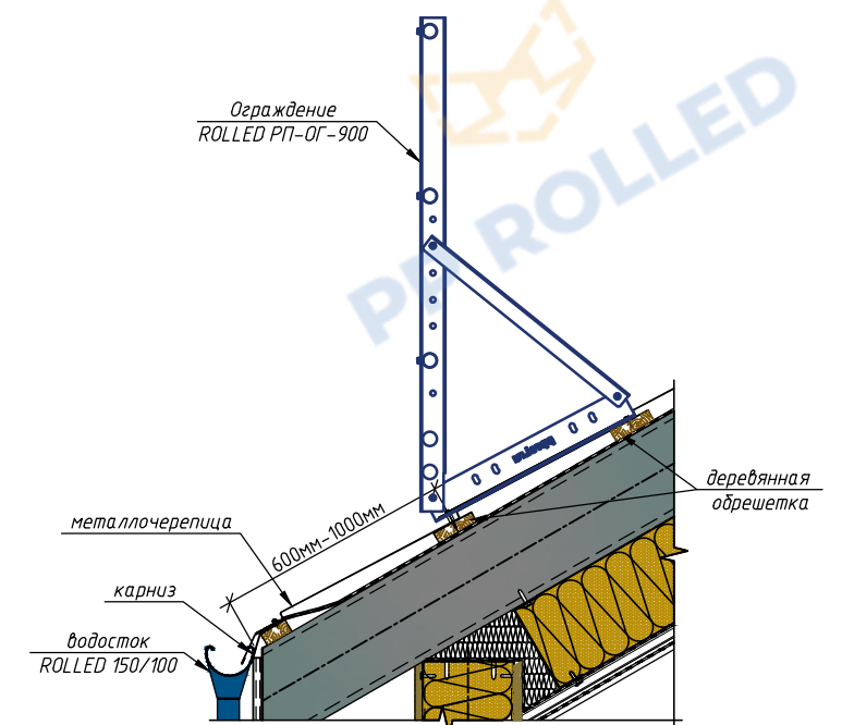
Типовой узел крепления ограждения на металлочерепицу
