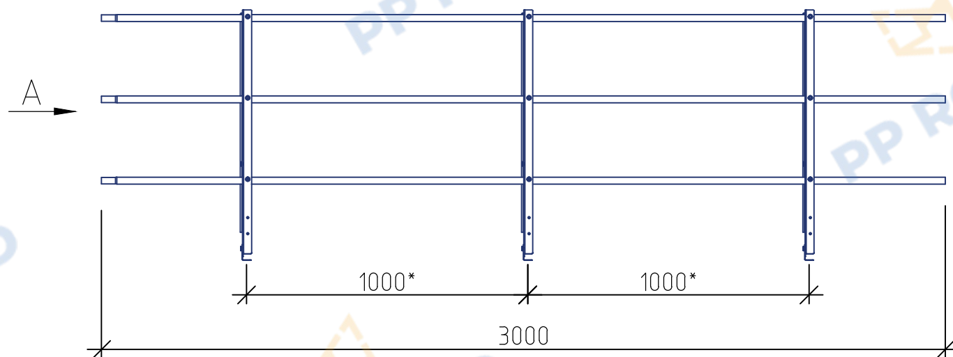
Ограждение РП-ОГ-900 (L=3000мм) PP ROLLED
