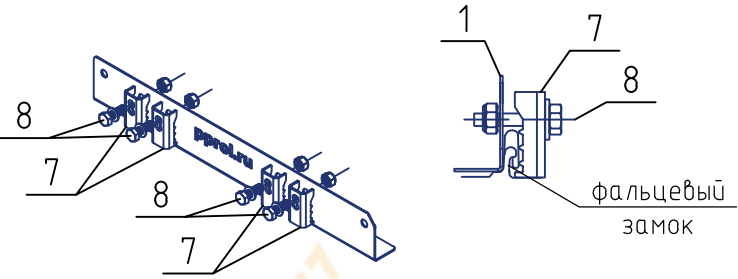
Опора РП-ОГ в сборе
