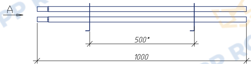
Снегозадержатель РП-СН-25-1,5 (2 опоры)
