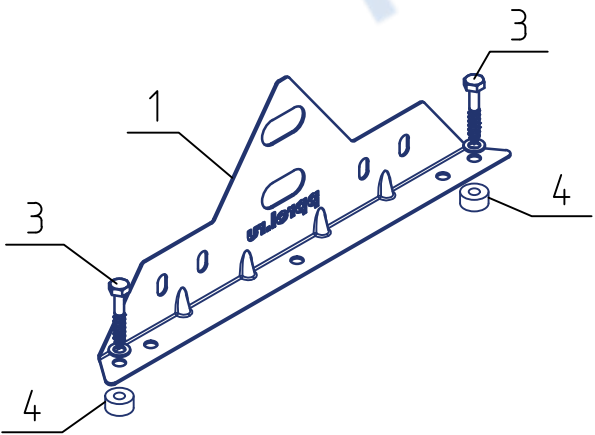
Крепление опоры
