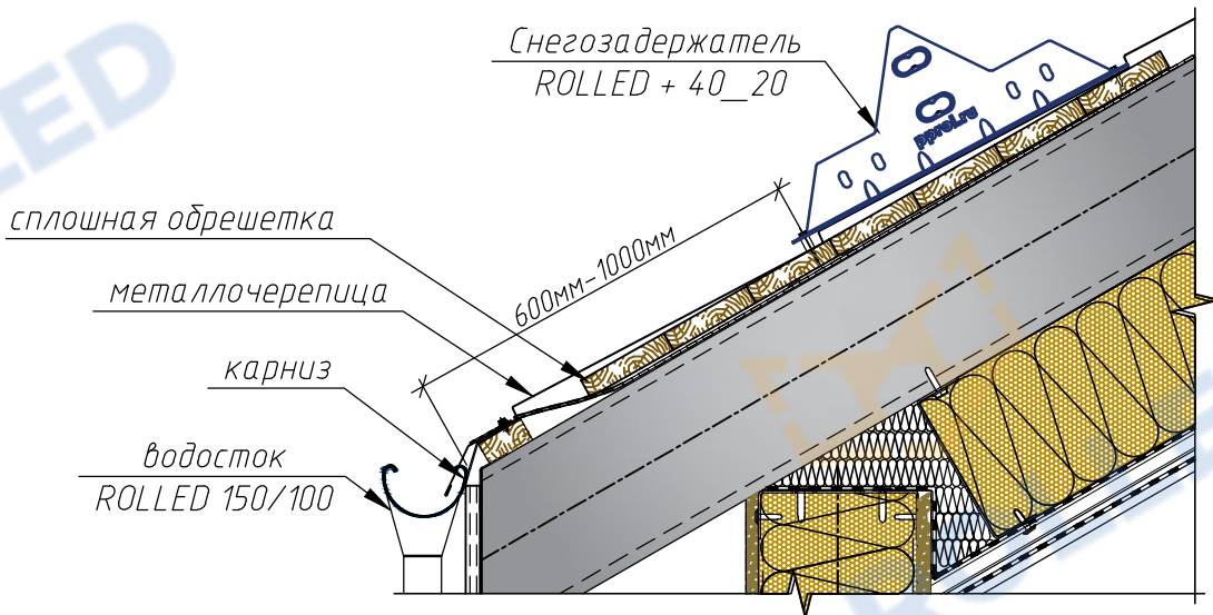
Типовой узел крепления снегозадержателя на металлочерепицу
