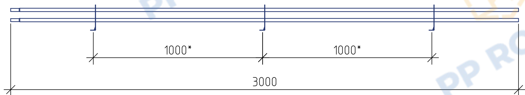
Снегозадержатель ROLLED+ 40_20-1,5 L=3000мм (3 опоры) PP ROLLED
