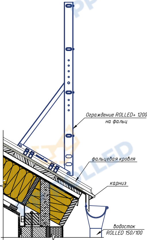
Типовой узел крепления ограждения на фальцевую кровлю
