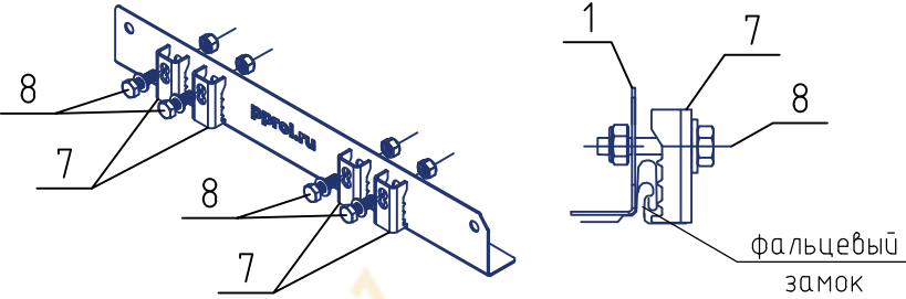
Опора РП-ОГ в сборе
