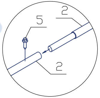
Узел крепления труб
