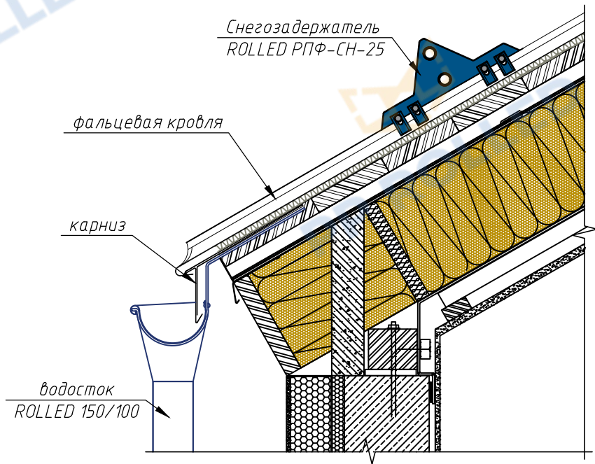
Типовой узел крепления снегозадержателя на фальцевую кровлю
