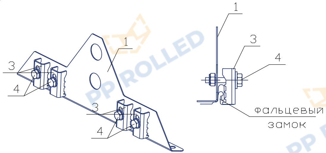
Опора РП-СН в сборе
