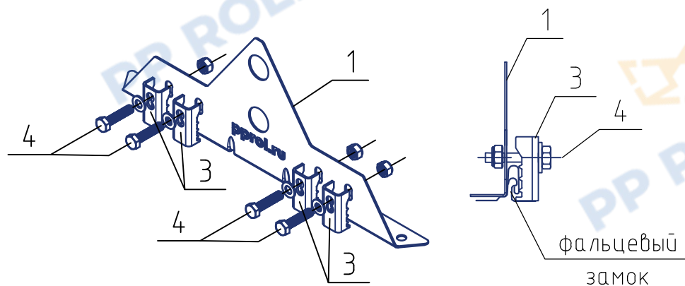
Крепление опоры
