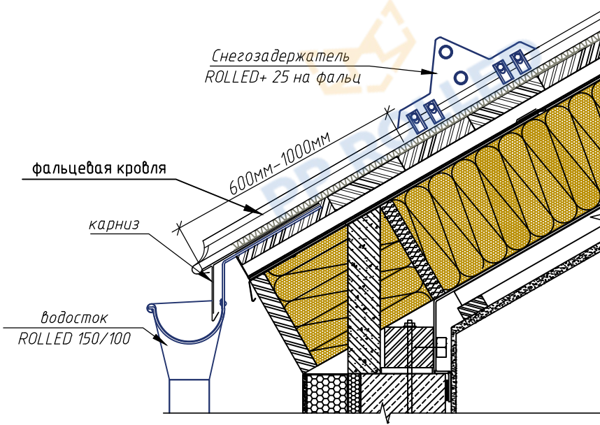
Типовой узел крепления снегозадержателя на фальцевую кровлю
