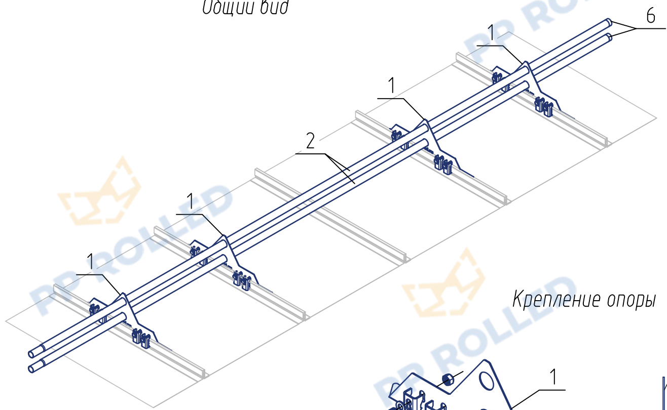
Общий вид
