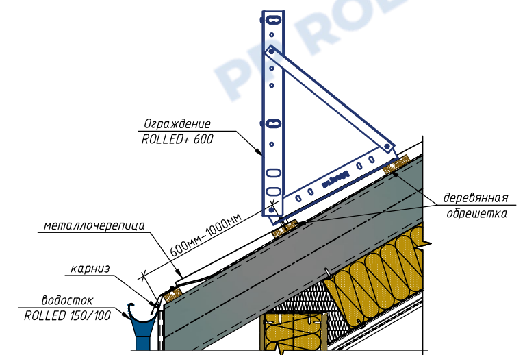
Типовой узел крепления ограждения на металлочерепицу
