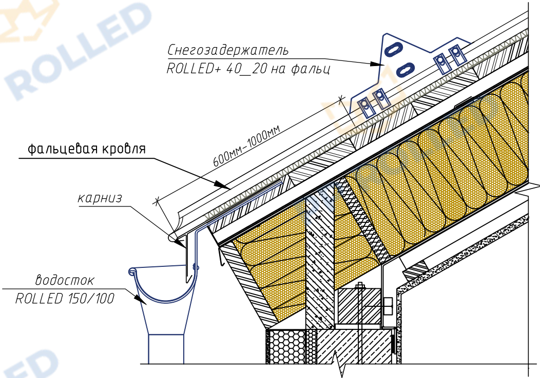
Типовой узел крепления снегозадержателя на фальцевую кровлю
