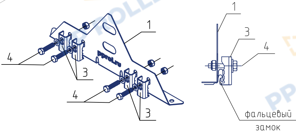
Крепление опоры
